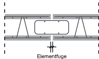
Horizontalschnitt Wand
